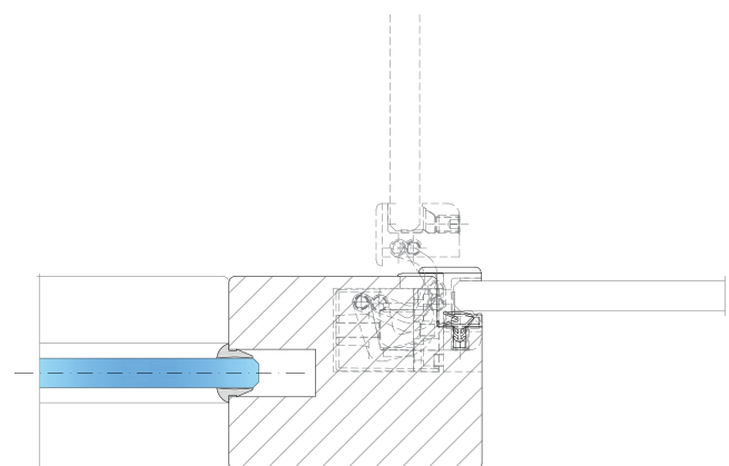
H81 ajtókeret | teliüveg ajtó | Tectus TE Glass | 32 dB-ig
