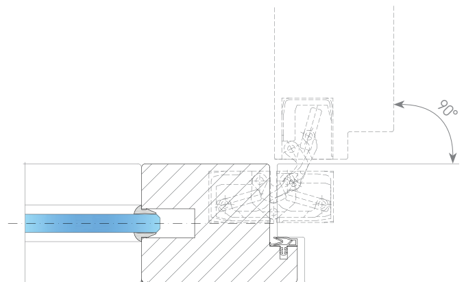
H80 ajtókeret | fa ajtó | Tectus TEG 310 | 37 dB-ig
