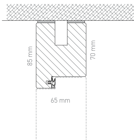
H80 ajtókeret | ajtókeret-áthidalás a mennyezetén
