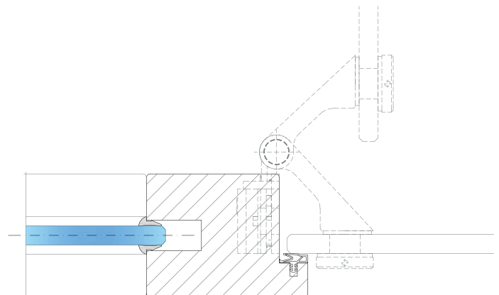
H80 ajtókeret | teliüveg | Just 3D | 32 dB-ig
